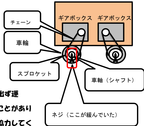
図1. 動力車の概略図
