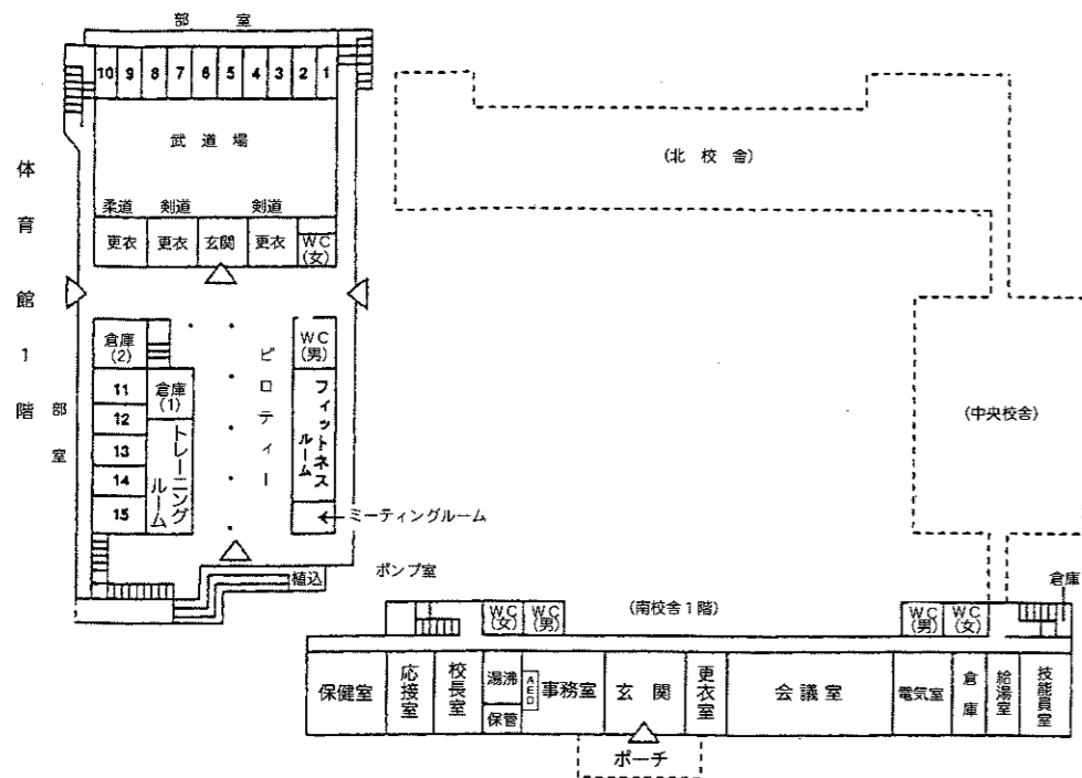
南校舎1階 平面図
