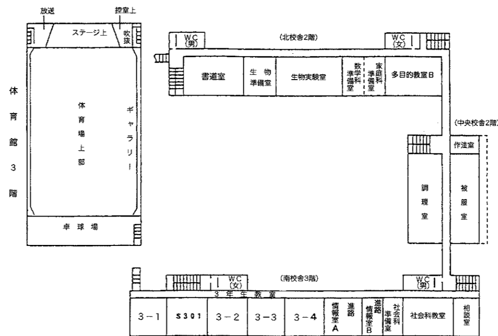
北校舎2階・南校舎3階 平面図
